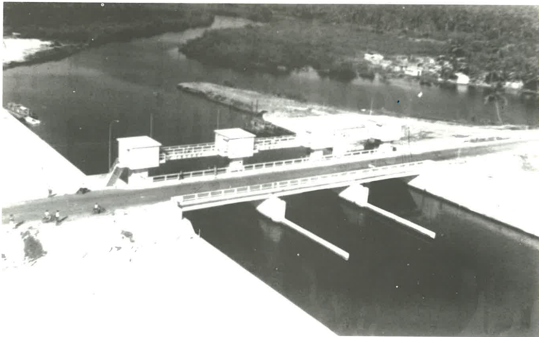
Dique de contención , Nagua.
